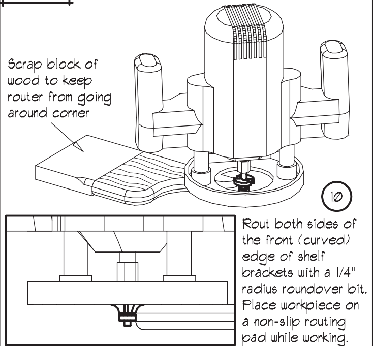
DIAG 8. ROUT BRACKET EDGE
